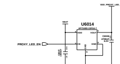
PROXY LDO
